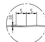
Деталь. А (2:1)
